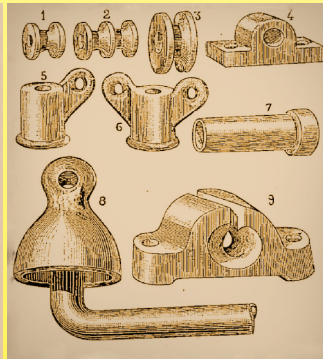
1885 год. Фарфоровые электроизоляторы (La physique moderne: l'électricité dans la maison, E. Hôpitalier)
