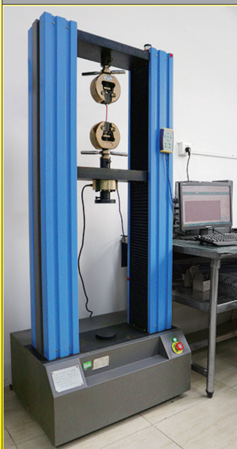
Испытательная установка для выполнения испытаний на отрыв
